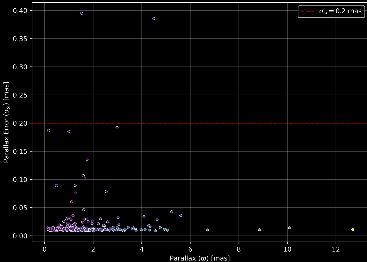
GALAH DR4 Field: [1056] Parallax Quality (n= 298)
