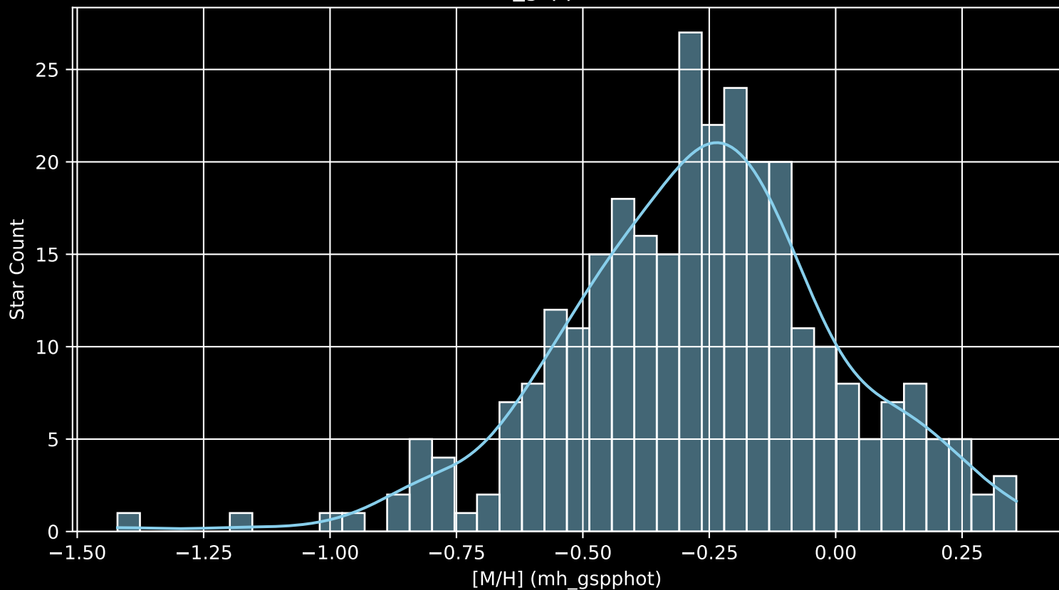
GALAH DR4 Field: [1056] [M/H] (mh_gspphot) (n= 297)
